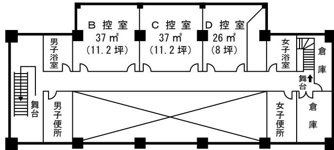
中2階控室その他平面図
