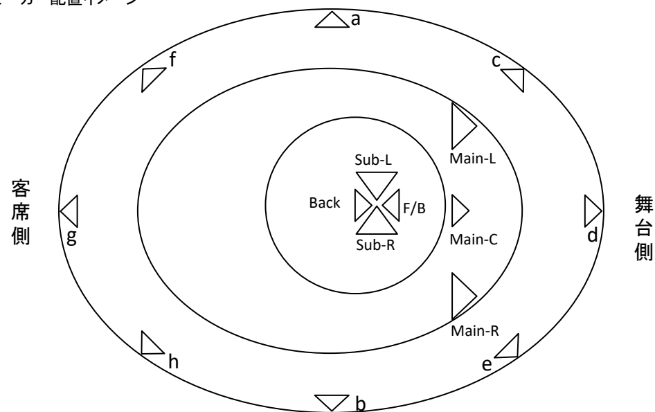
スピーカー配置イメージ
